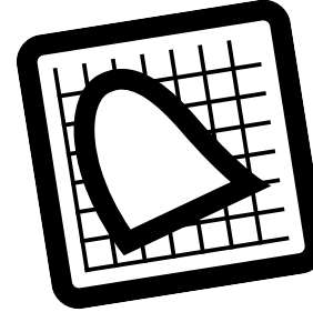
färgrymd
